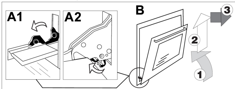
Skidanje stakla sa okna vrata
