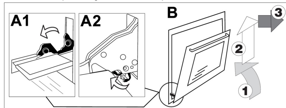
Вадење на стаклото на вратата
